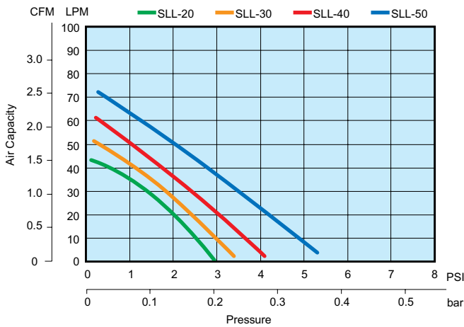
220V 50Hz
