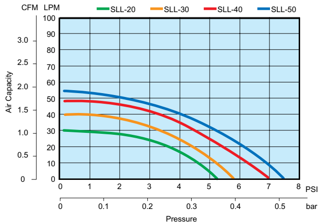
115V 60Hz
